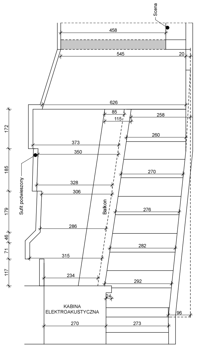
PRZEKRÓJ B-B
